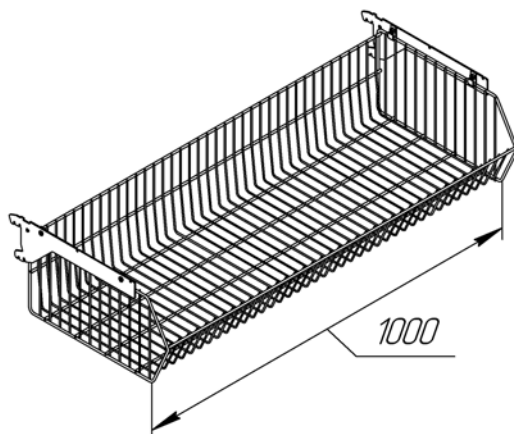
Комплект для корзины оцинкованной СК100.15.00.000СБ
