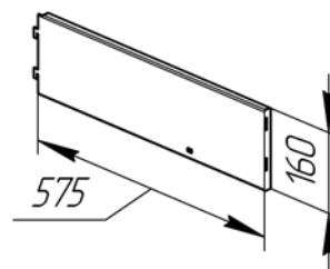
② Кронштейн фриза левый СК100.05.00.020
