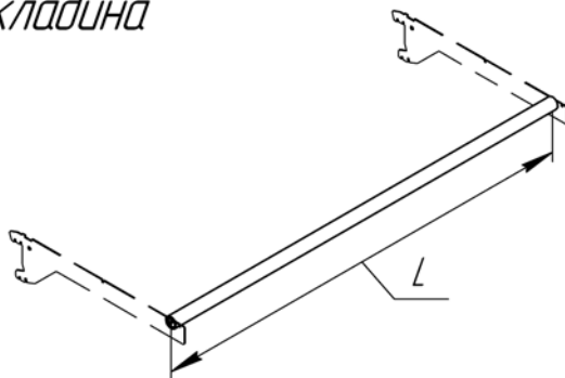
Держатель
