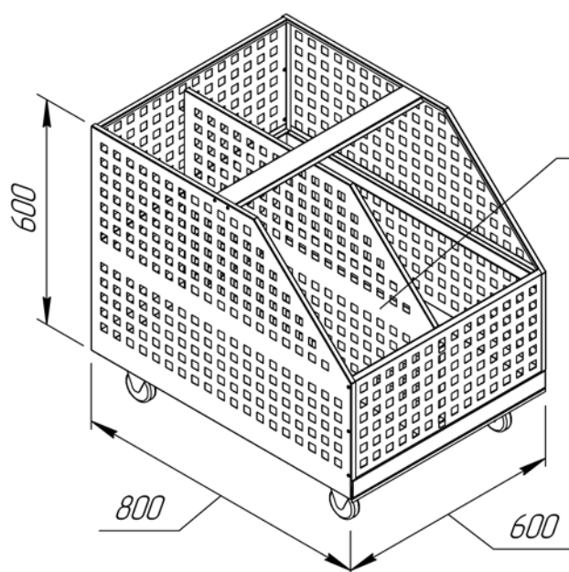
Перегорodka КО.05.00.000СБ *
