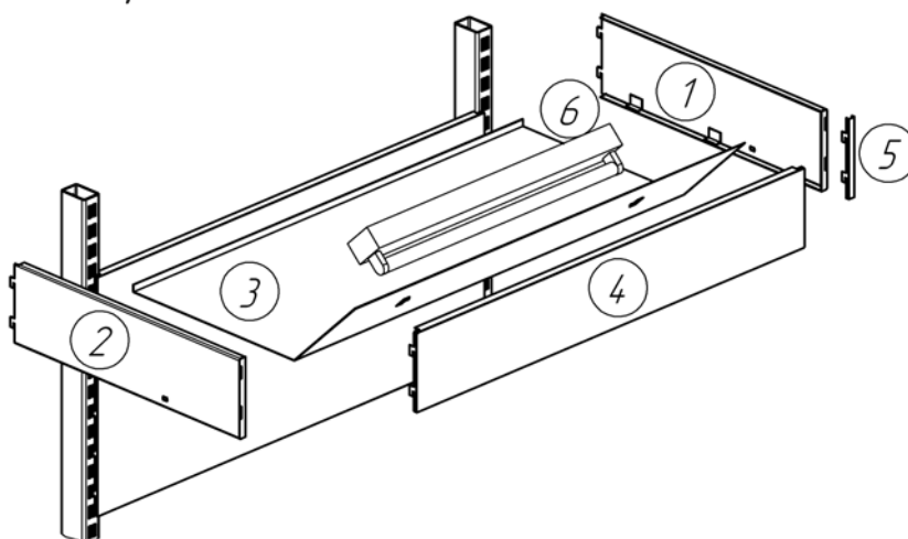
① Кронштейн фриза правый СК100.05.00.010
