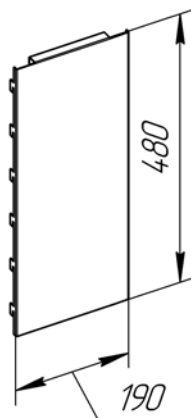
⑫ Панель задняя СМУН.00.00.001
