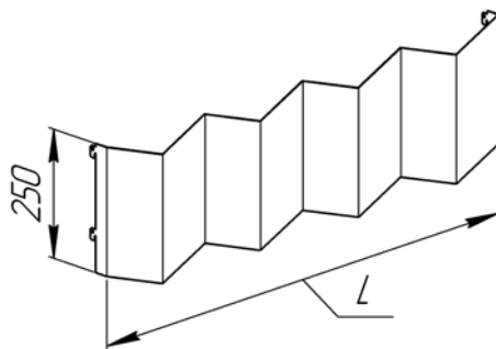
Полка "гармошка"
