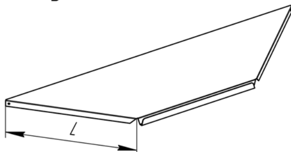
⑪ Полка угловая
