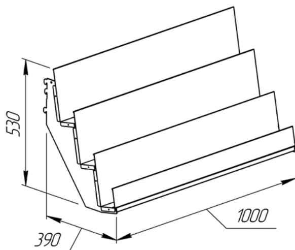
Полка книжная СК100.38.00.000СБ
