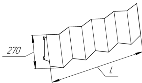
Полка "гармошка" наклонная
