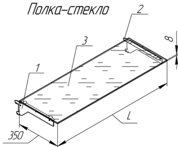
Полка-стекло
