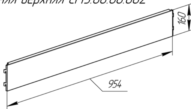
⑨ Панель задняя верхняя СМУ.00.00.002
