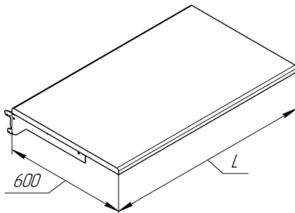
Полка-постформинг
