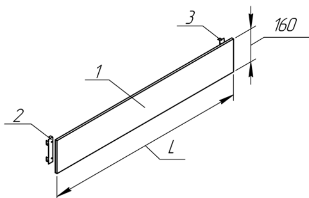
Панель фриза ДСП
